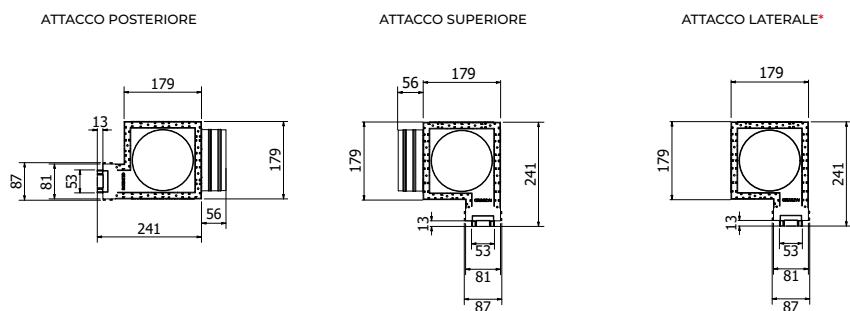
DIMENSIONALI PS2F H50 - INSTALLAZIONE CARTONGESSO
